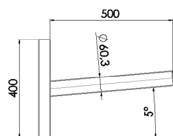
Crosse murale A réf 777002 GALVA B réf 770057 RAL 7012
